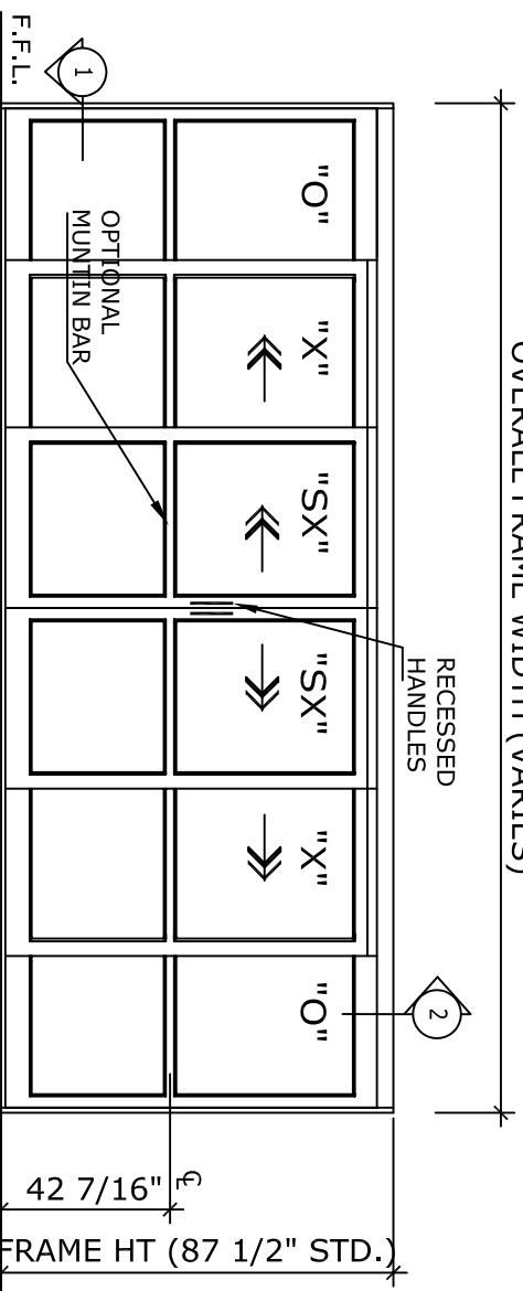
DOOR ELEVATION
